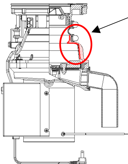
【図1：ディスポーザ構造図】
